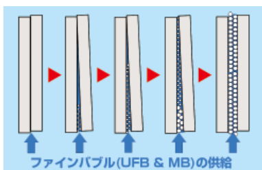
【上】ファインバブル水中の太陽電池シリコンウェハースのインゴットの様子。密着した薄膜ウェハースが、時間が経つにつれ（写真の右側に向かって）分離していくのがわかる。／【下】ウェハース分離のプロセス。ウェハースの間隙には、UFB から MB へと次第に大きなバブルが浸透し、ウェハース 1 枚 1 枚を分離していく。
